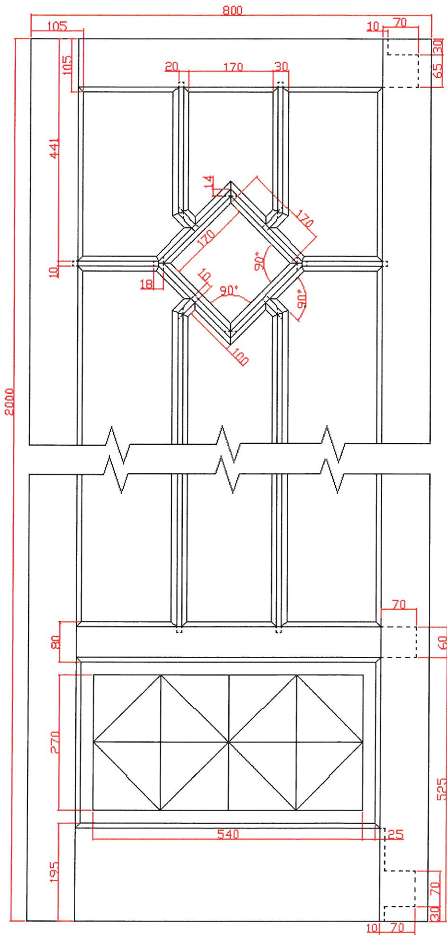
konkursa nominācijai Galdnieks (H x P x Dz = 2000 x 800 x 40; materiāls: bērza vai melnalkšņa masīvkoksnes sagataves).
